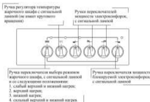
Рис. 9. Передняя панель плиты ЭП 411СТ
