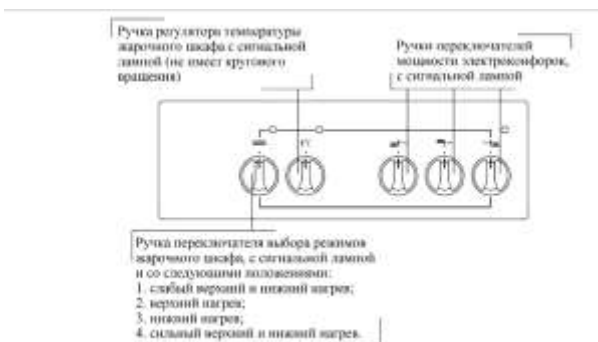
Рис. 8. Передняя панель плиты ЭП 301СТ
