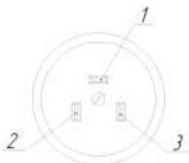
Рис. 1. Подключение розетки
