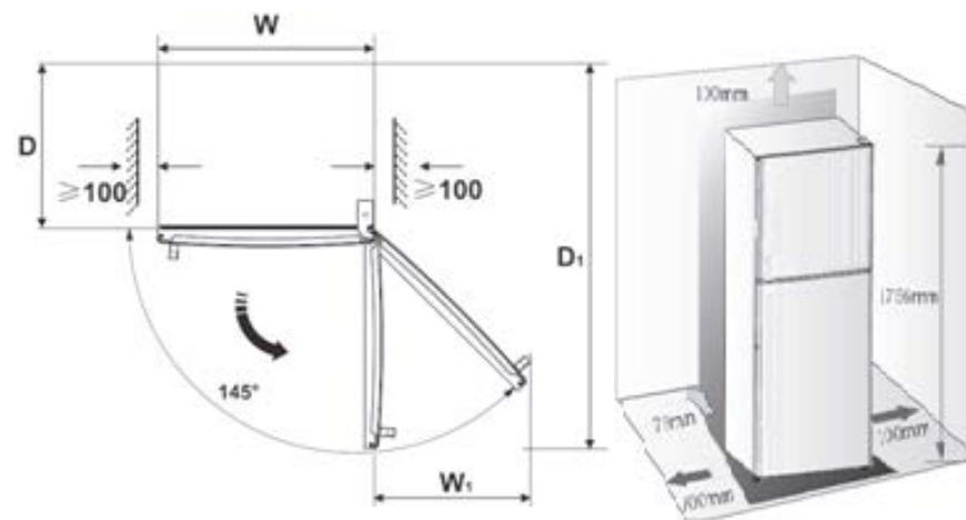
Рисунок-схема рекомендуемого размещения холодильника
