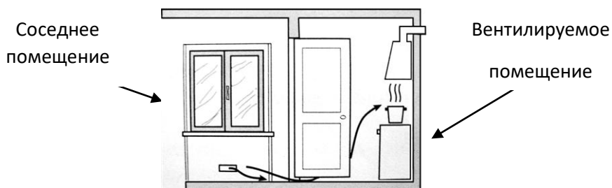
Рис. В Косвенный приток воздуха с увеличением вентиляционной щели между окном и полом
