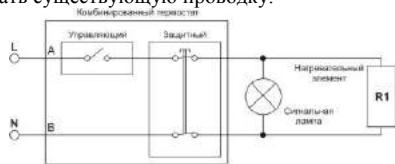
Рис. 8. Схема электрическая для моделей E-series, O'Prio, EGO, O'Prio+
