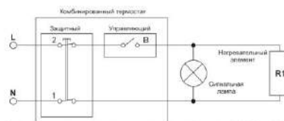
Рис.9. Схема электрическая для моделей Steatite (N3CM, N4C (E)).
