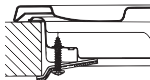
Poziția clemei pentru sus H=40mm
