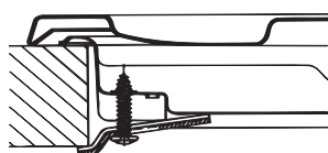
Монтаж крюка для опорных брусьев H=40\text{mm}
