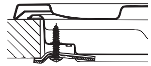
Poziția clemei pentru sus H=30mm
