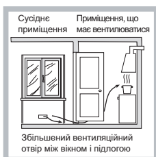
Приклади вентиляційних отворів для відводу повітря з продуктами горіння.
