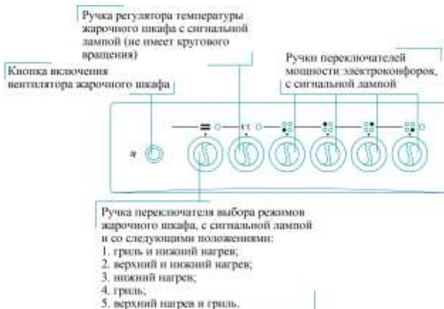
Рис. 7 Передняя панель плиты ЭПС404 MS
