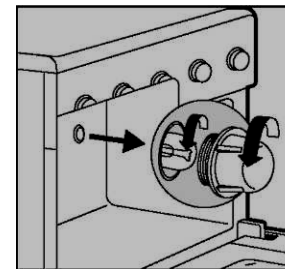
Рисунок 13 – Замена лампы освещения
