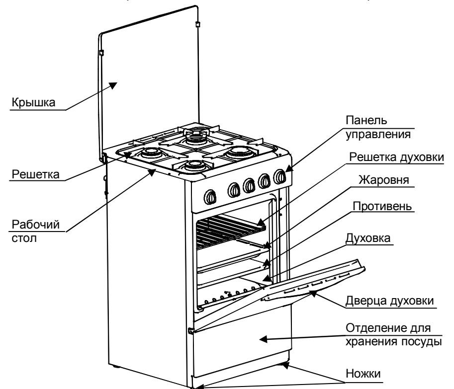
Рисунок 1 – Устройство плиты
