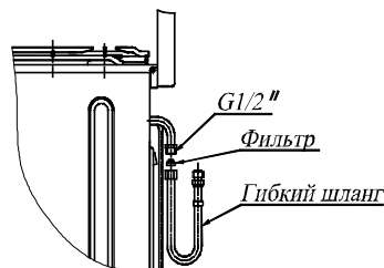
Рисунок 8 – Схема подключения гибкого шланга прямым соединением
