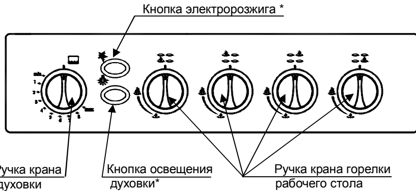
Рисунок 3 – Панель управления
