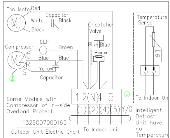
Наружный блок моделей RAS/RAC-24AX,30AX,36AX
