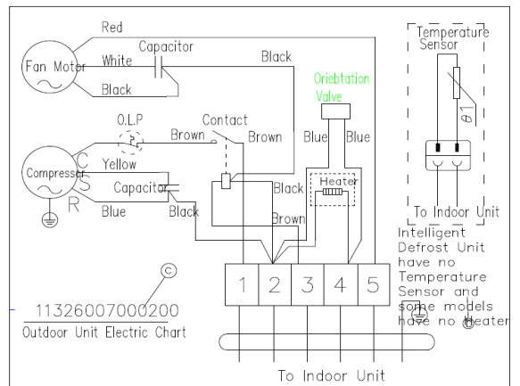
Наружный блок моделей RAS/RAC-24AX,30AX,36AX
