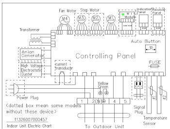
Внутренний блок моделей RAS/RAC-24AX, 30AX, 36AX
