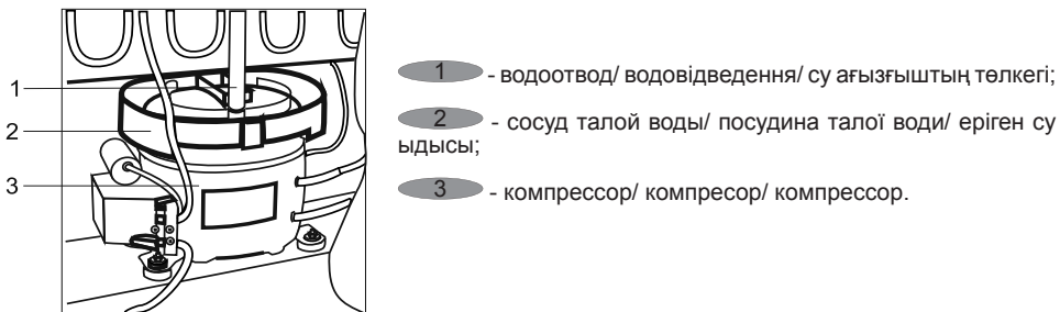
Рисунок Б.4 - Схема отвода талой воды из холодильной камеры Рисунок Б.4 - Схема відведення талої води з холодильної камери Б.4-сурет - Тоңазытқыш камерадан еріген судың ағу сызбанұсқасы
