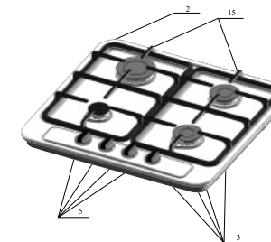
Рисунок 6 Встраиваемый блок (тип ВГ стиль М) Встраиваемый блок – это специальное устройство для приготовления пищи за счет образования тепла от сгорания газа в газовых горелках. Горелки расположены на рабочем столе плиты. Управление работой газовых горелок осуществляется кранами. Для розжига горелок используется интегрированный розжиг. Для горения горелки используется воздух помещения. Специальное устройство для отвода продуктов сгорания газа не предусмотрено. В зависимости от стиля, поверхность встраиваемого блока может быть эмалированной, стеклянной, из нержавеющей стали.
