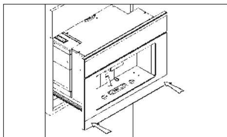
Fig. 7.8 Empurrar a máquina no interior do alojamento e exercitar uma leve força até ouvir o "CLICK!" de bloqueio.
