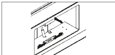
Fig. 7.2 Premere le leve di sblocco situate sotto la bacinella raccogli gocce e tirare la macchina verso di se agendo come in figura.
