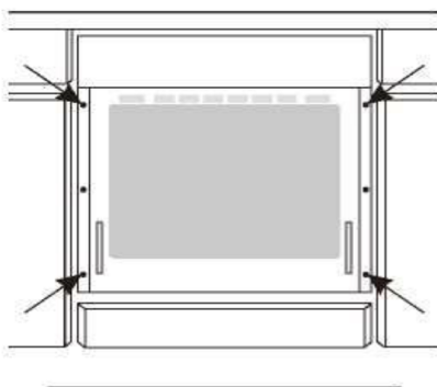
Габариты изделия
