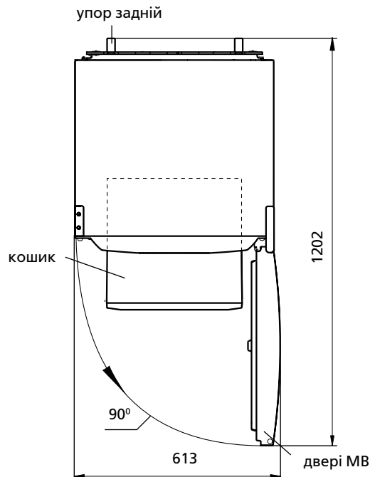
Рисунок 2 – Холодильник (вигляд зверху)
