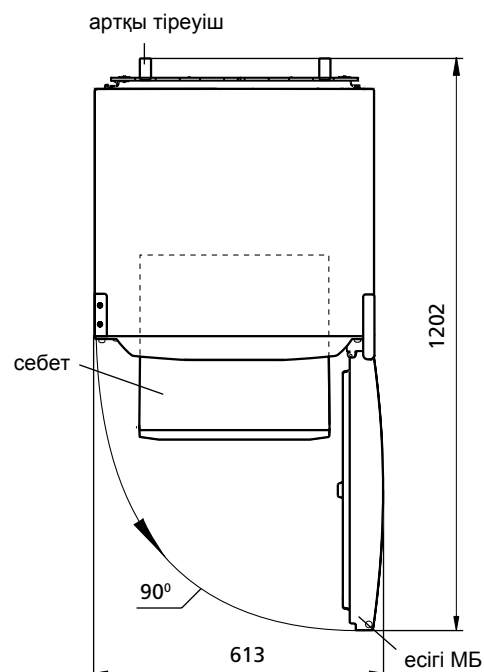
Сурет 2 – Тоңазытқыш (үстінен қарағанда)
