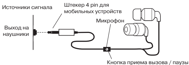
Рис. 1. Схема подключения
