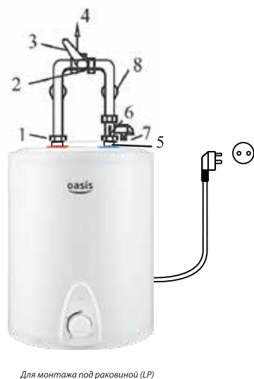
Для монтажа под раковиной (LP)
